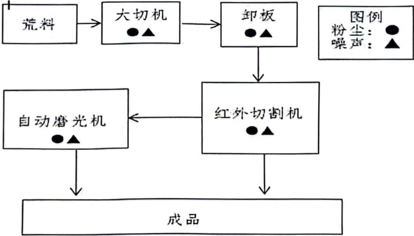
图 4-1 生产工艺流程图
